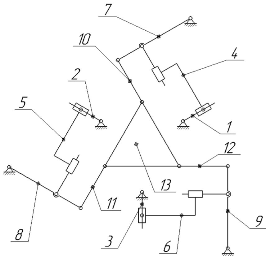
Рисунок 2.19 - Синтезированный многоконтурный механизм с тремя степенями свободы: 1,2,3 – кривошипы, выполненные с возможностью регулировки длины; 4,5,6 – шатуны, выполненные с возможностью регулировки длины; 7,8,9 – коромысла; 10,11,12 – промежуточные шатуны; 13 – выходное звено (платформа)
