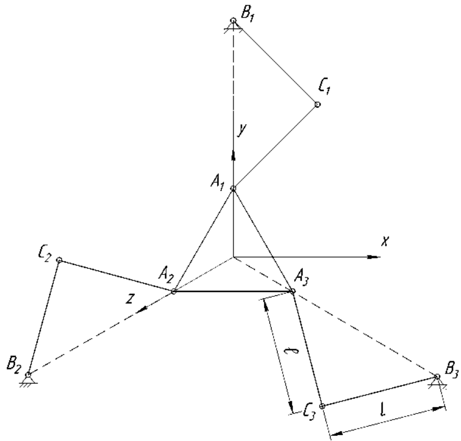
Рисунок 4.1 – Исследуемый механизм: A_k, B_k, C_k – кинематические пары; k = 1, 2, 3
