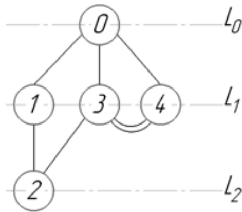
Рисунок 2.8 – Граф синтезированного механизма
