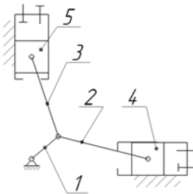
Рисунок 2.7 - Синтезированный механизм для преобразования вращательного движения в возвратно-поступательное с одной степенью свободы:
