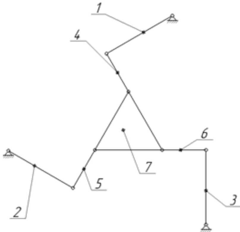
Рисунок 2.17 - Синтезированный двухконтурный механизм с тремя степенями свободы: 1,2,3 – коромысла; 4,5,6 – шатуны; 7 – выходное звено (платформа)
