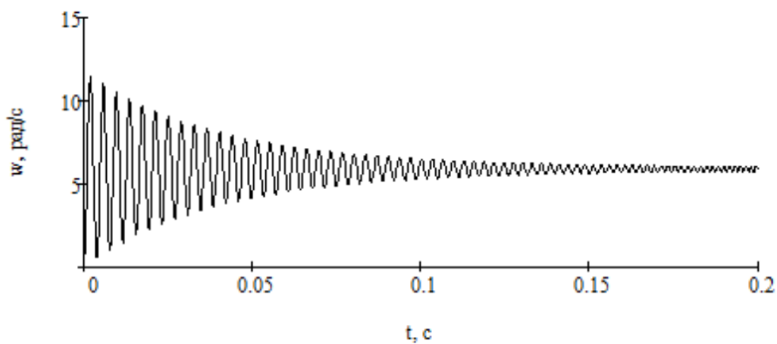
Рисунок 4.4 – Изменение угловой скорости вращения электродвигателя
