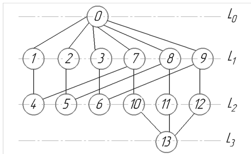
Рисунок 2.18 - Граф механизма
