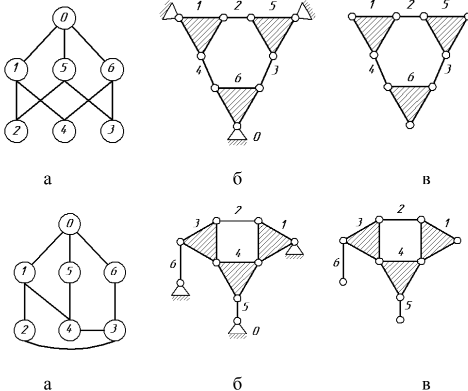
Рисунок 2.4: а - граф фермы; б – ферма структурной группы, в – синтезированная структурная группа
