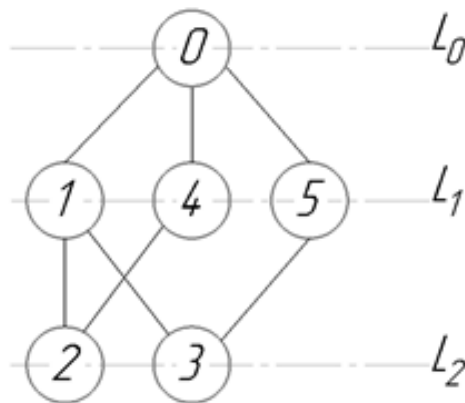
Рисунок 2.6 - Граф механизма
