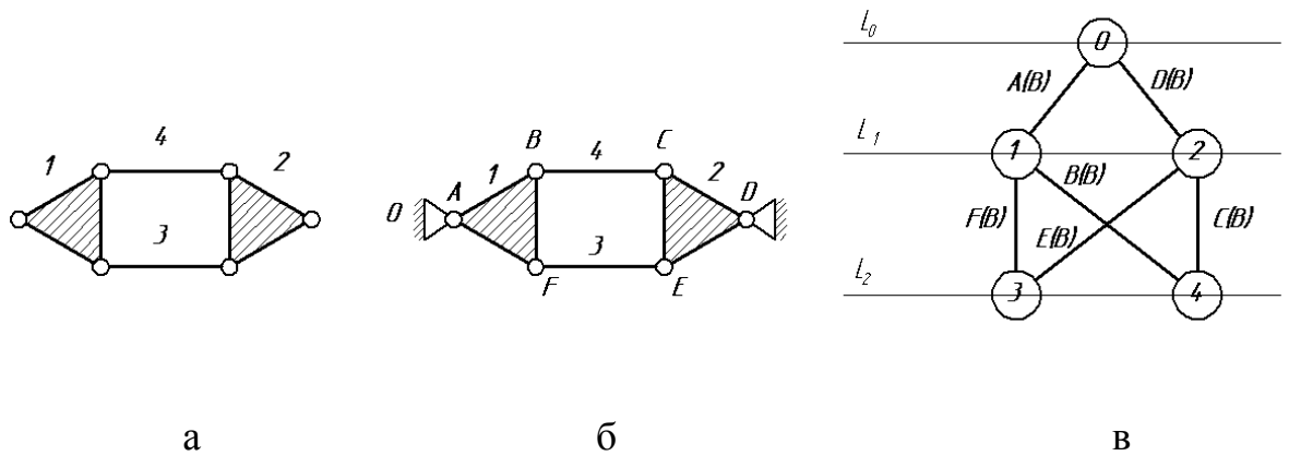
Рисунок 2.1: а – структурная группа; б – ферма на основе структурной группы; в – граф фермы
