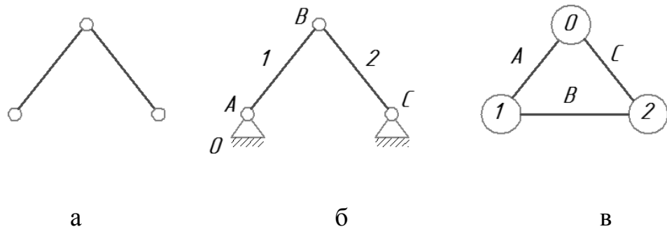
Рисунок 2.3: а – двухповодковая диада; б – ферма на основе диады; в – граф фермы
