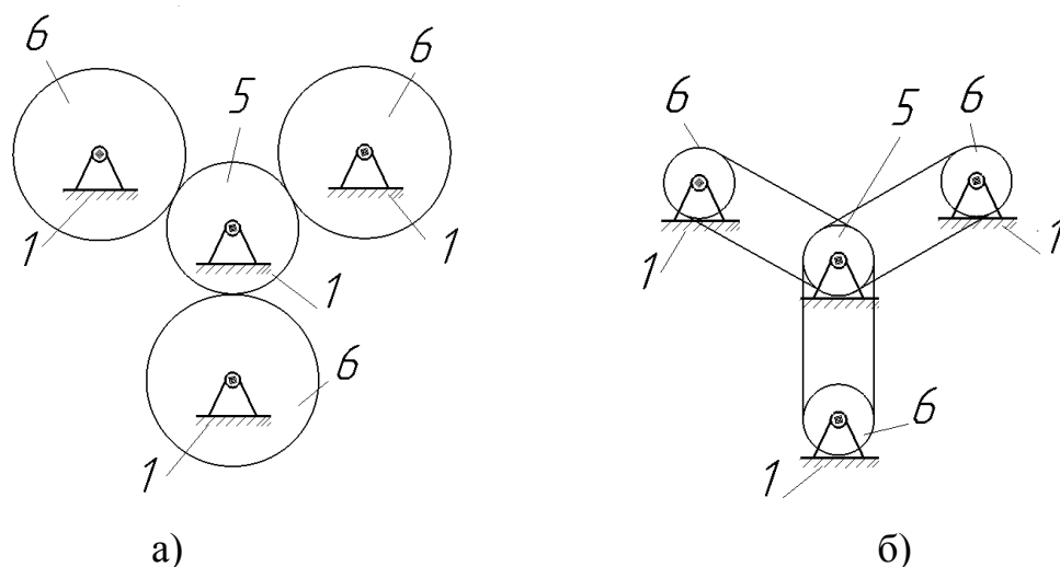
Рисунок 3.2 – Сопряжения двигателя с входными звеньями: а) зубчатым зацеплением; б) ременной передачей
